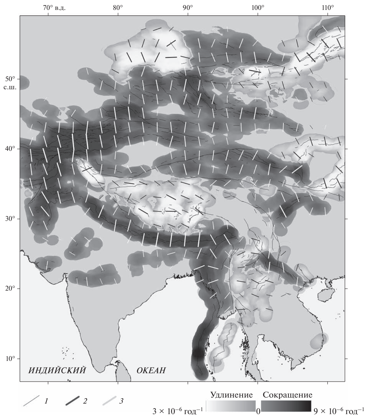
Рис. 3. Величины деформации максимального латерального удлинения и укорочения. Центральной Азии, 10^{-6} 1/год (шкала оттенков серого).
