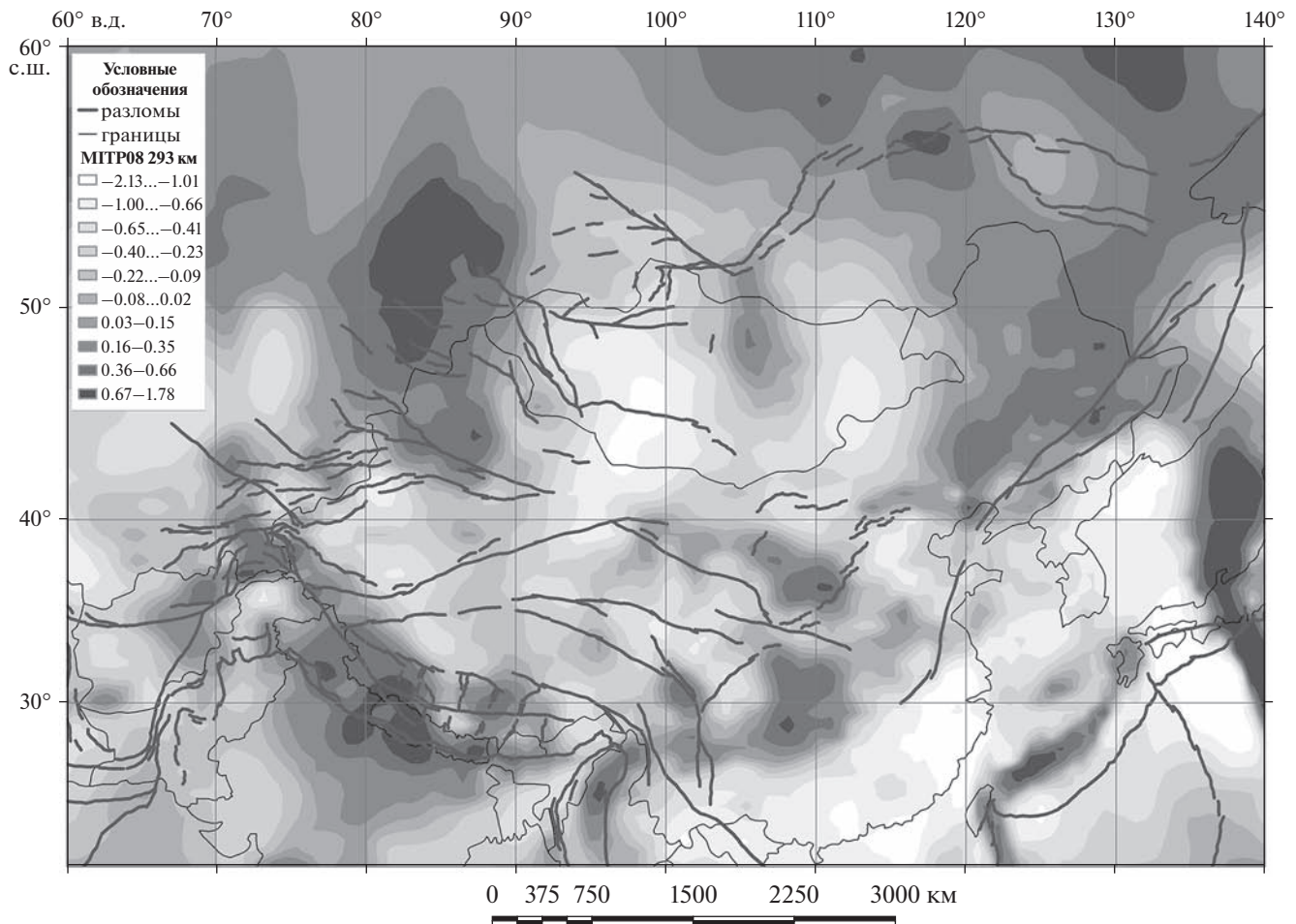
Рис. 7. Схема строения верхней мантии Центральной Азии на глубине 293 км ниже уровня моря. Представлены отклонения скоростей продольных волн от стандартных для этой глубины значений по данным сейсмографической модели MIT-P08 [47].
