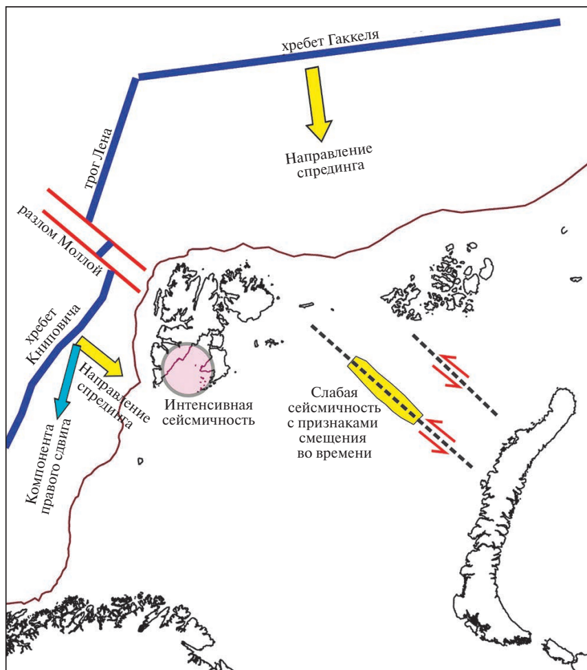
Рис. 8. Схема геодинамики района исследований с элементами, необходимыми для интерпретации тектоники внутри шельфа Баренцева моря. Размеры векторов воздействия на плиту имеют условный характер.
