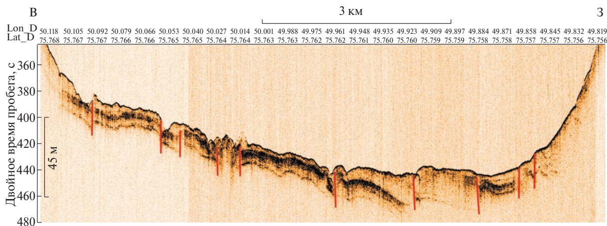
Рис. 4. Фрагмент сейсмоакустического разреза АВР51_2209212244, полученного высокочастотным профилографом ParaSound P-35 в 51-м рейсе НИС “Академик Борис Петров” (октябрь–ноябрь 2022 г., ИО РАН, ГИН РАН) в центральной части Баренцева моря, пересекающий зону сдвиговых дислокаций северо-западной ориентации. Красными линиями показаны сбросы и взбросы, нарушающие верхнюю часть разреза и выходящие к поверхности дна. Положение фрагмента показано на рис. 1.
