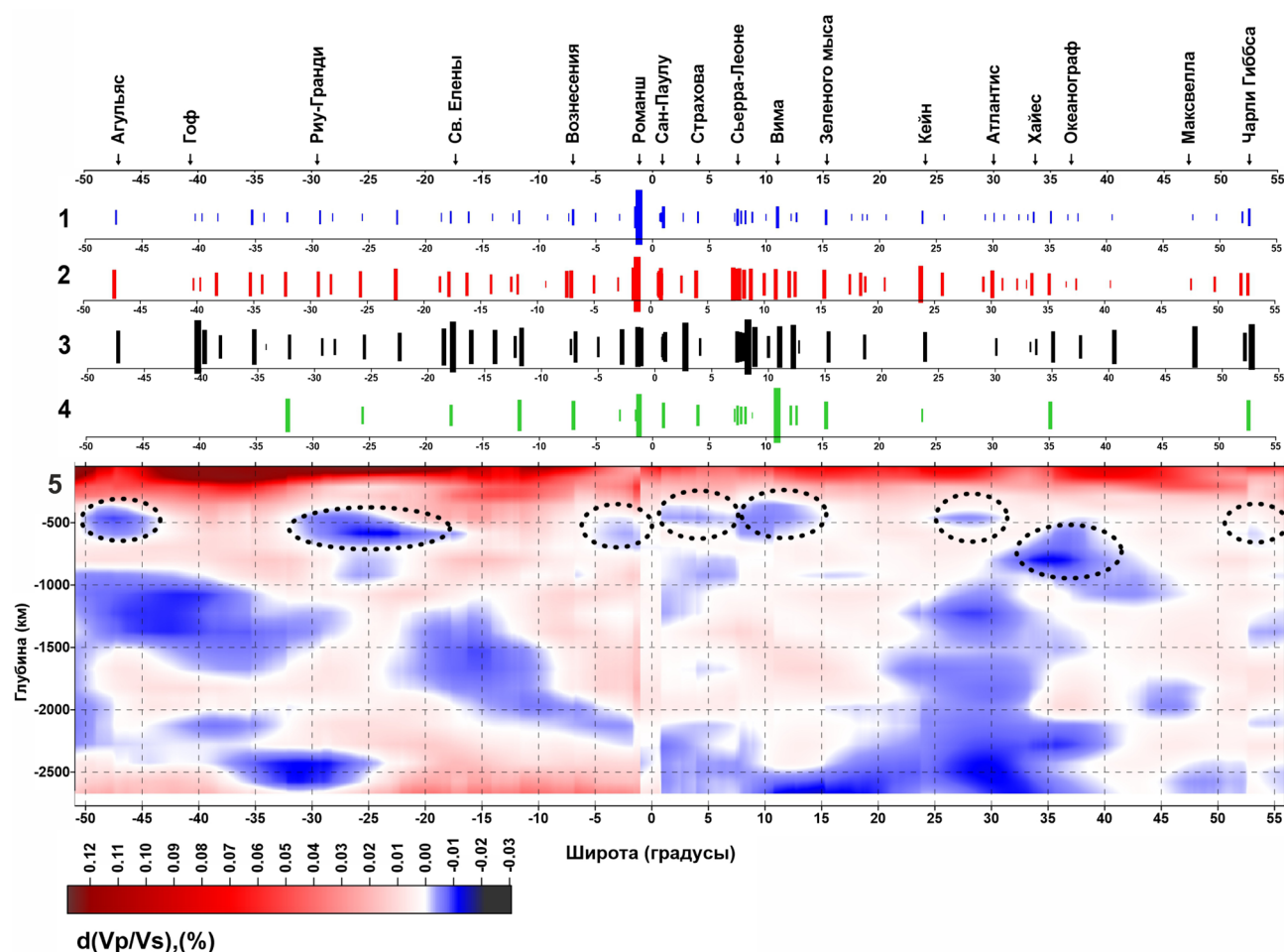
Рис. 3. Корреляция характеристик морфометрических параметров трансформных разломов САХ, рассматриваемых в работе (гр. 1–4) и разрез вариации отношения V_p/V_s . Графики сопоставляемых характеристик: 1 — положения зон смещения трансформных разломов с размером символа, линейно пропорциональным длине активной части (от 10 до 950 км); 2 — положения зон смещения трансформных разломов с размером символа, линейно пропорциональным максимальной глубине в пределах трансформной долины (от 3100 до 7800 м); 3 — положения зон смещения трансформных разломов с морфологически четко выраженной трансформной долиной с размером символа, линейно пропорциональным ширине трансформной долины (от 3 до 36 км); 4 — положения зон смещения трансформных разломов с морфологически четко выраженным приразломным хребтом с размером символа, обратно пропорциональным минимальной глубине приразломного хребта (от 500 до 3000 м); 5 — вариации отношения V_p/V_s , рассчитанные по сейсмотомографическим данным для Р и S, пунктирными кругами обозначены «холодные» аномалии верхней мантии (Соколов, 2016).
