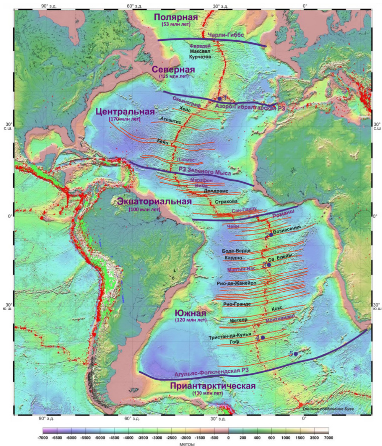
Рис. 1. Распределение разломных зон в пределах разных морфотектонических провинций Атлантического океана по (Мирлин, Сушевская, 1992; Мировой..., 2013). Синими линиями отмечены разломы, являющиеся границами между морфотектоническими провинциями (в скобках указан возраст начала раскрытия), красными точками — эпицентры землетрясений, синими кругами выделены «горячие точки», упомянутые в тексте. Цветом выделены названия разломов, использовавшиеся при анализе батиметрических данных. Горячие точки: 1 — Азорская, 2 — Вознесения, 3 — Св. Елены, 4 — Гоф, 5 — Дискавери.
