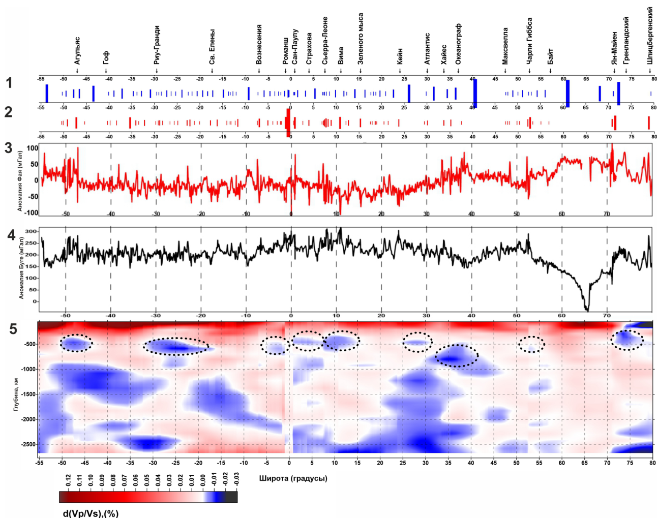
Рис. 2. Корреляция характеристик структурных элементов САХ (гр. 1–4) и разрез вариации отношения V_p/V_s . Графики сопоставляемых характеристик: 1 — центры сегментов САХ с размером символа, линейно пропорциональным длине сегментов (от 18 до 1186 км) и названия основных разломных зон, пересекающих САХ; 2 — положения зон смещения трансформных разломов с размером символа, линейно пропорциональным длине активной части (от 10 до 750 км); 3 — значения гравитационных аномалий в свободном воздухе (мГал); 4 — значения аномалий Буге (мГал); 5 — вариации отношения V_p/V_s , рассчитанные по сейсмо tomографическим данным для Р и S, пунктирными кругами обозначены «холодные» аномалии верхней мантии (Соколов, 2016).
